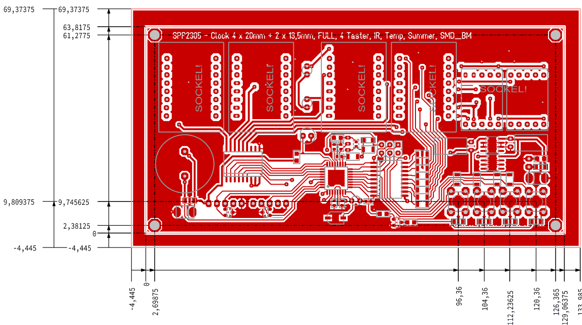
Abbildung 2: Beschreibung zum Einbau (Abmessungen) des Moduls SPP2305.4
