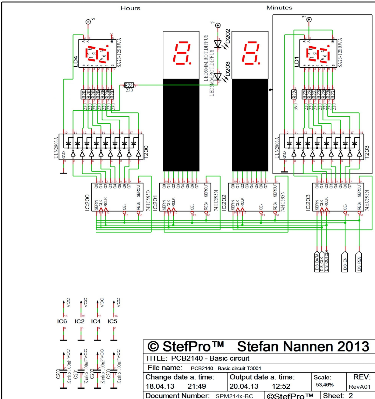
Abbildung 3: Grundschtung vom SPM2244P Teil 2
