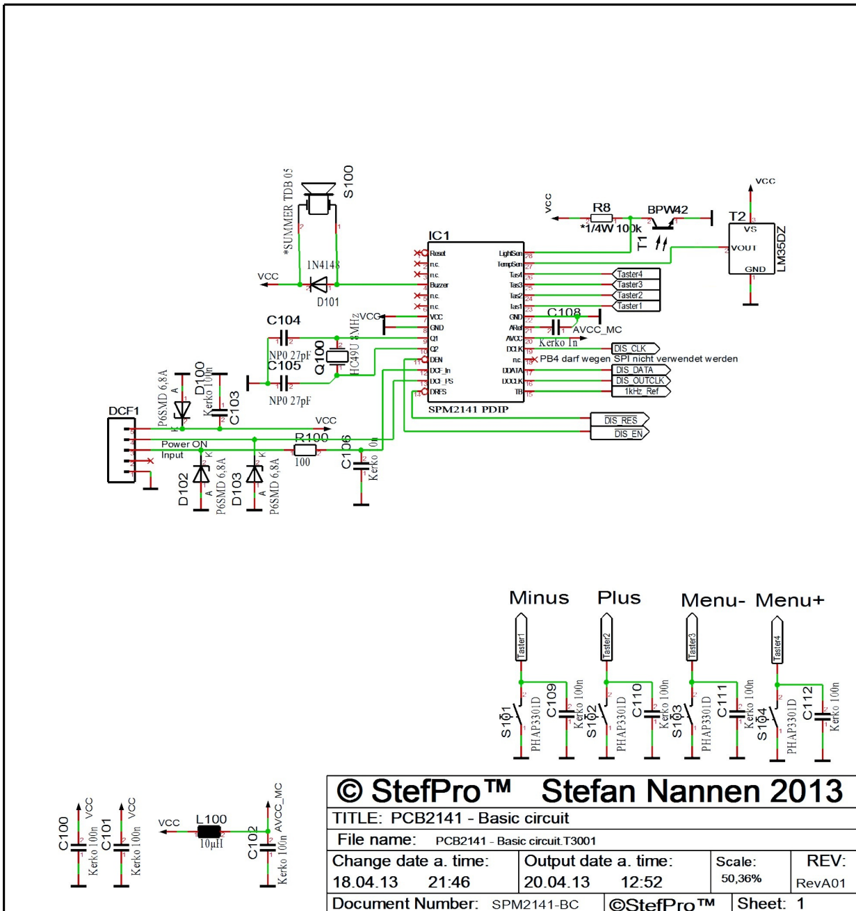
Abbildung 2: Grundschtaltung vom SPM2241P Teil 1
