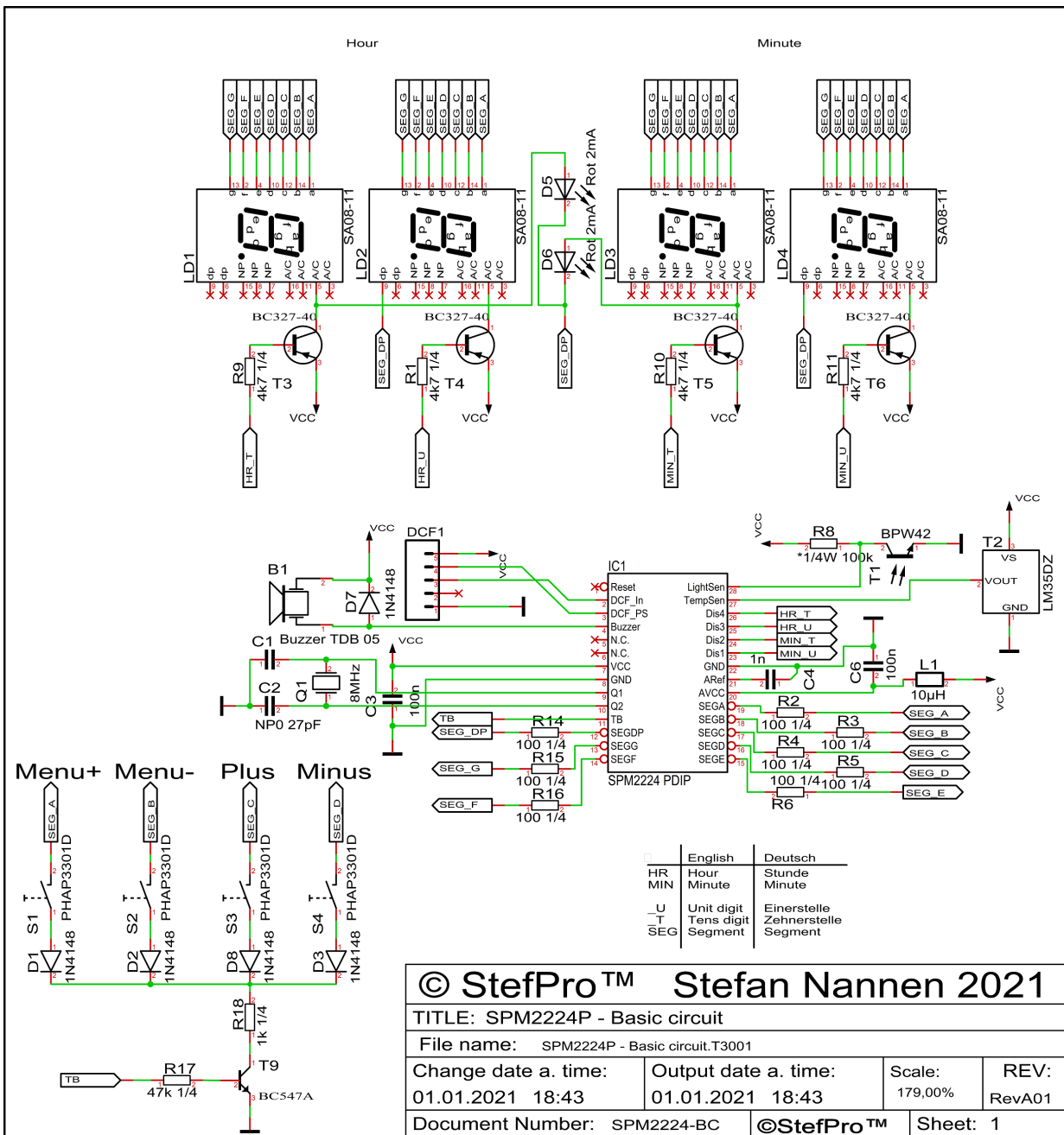
Abbildung 2: Grundschtaltung vom SPM2224P
