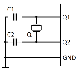
Abbildung 1: Anschluss des Quarzes
