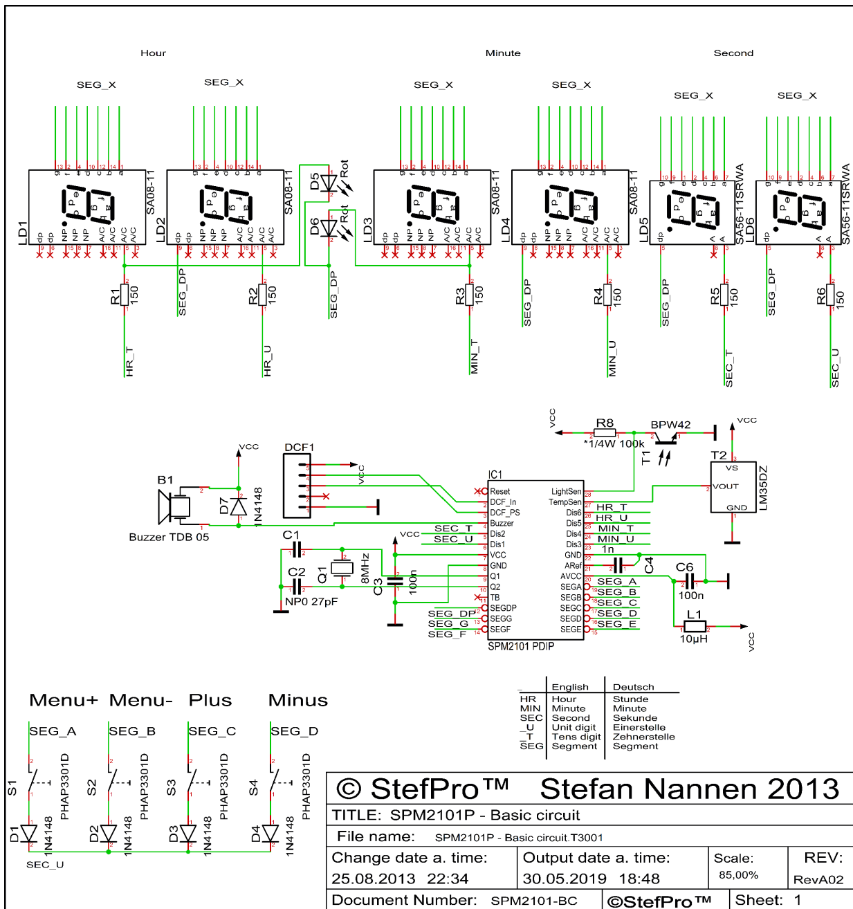
Abbildung 2: Grundschtaltung vom SPM2201P
