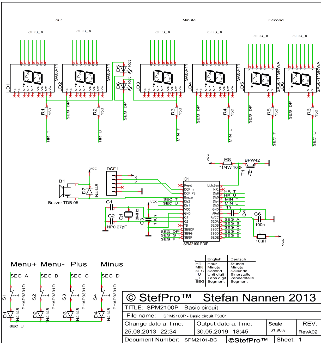
Abbildung 2: Grundschtaltung vom SPM2200P
