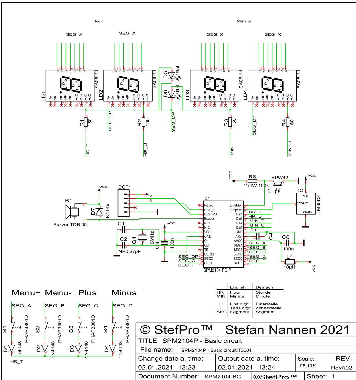
Abbildung 2: Grundschtaltung vom SPM2104P
