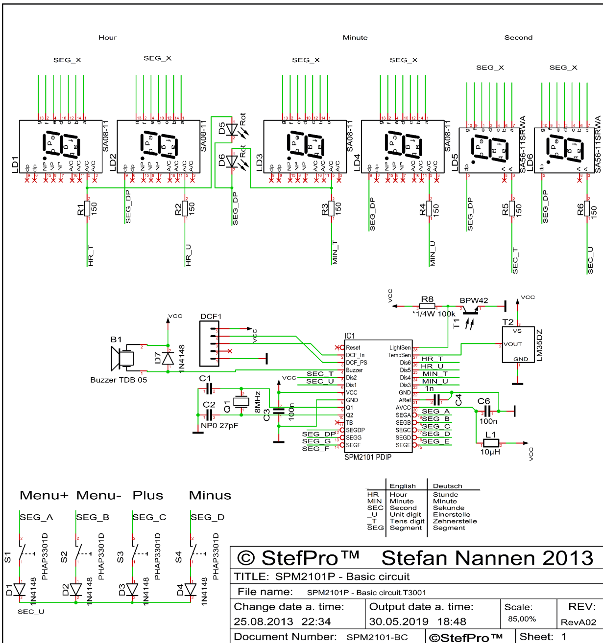
Abbildung 2: Grundschtaltung vom SPM2101P
