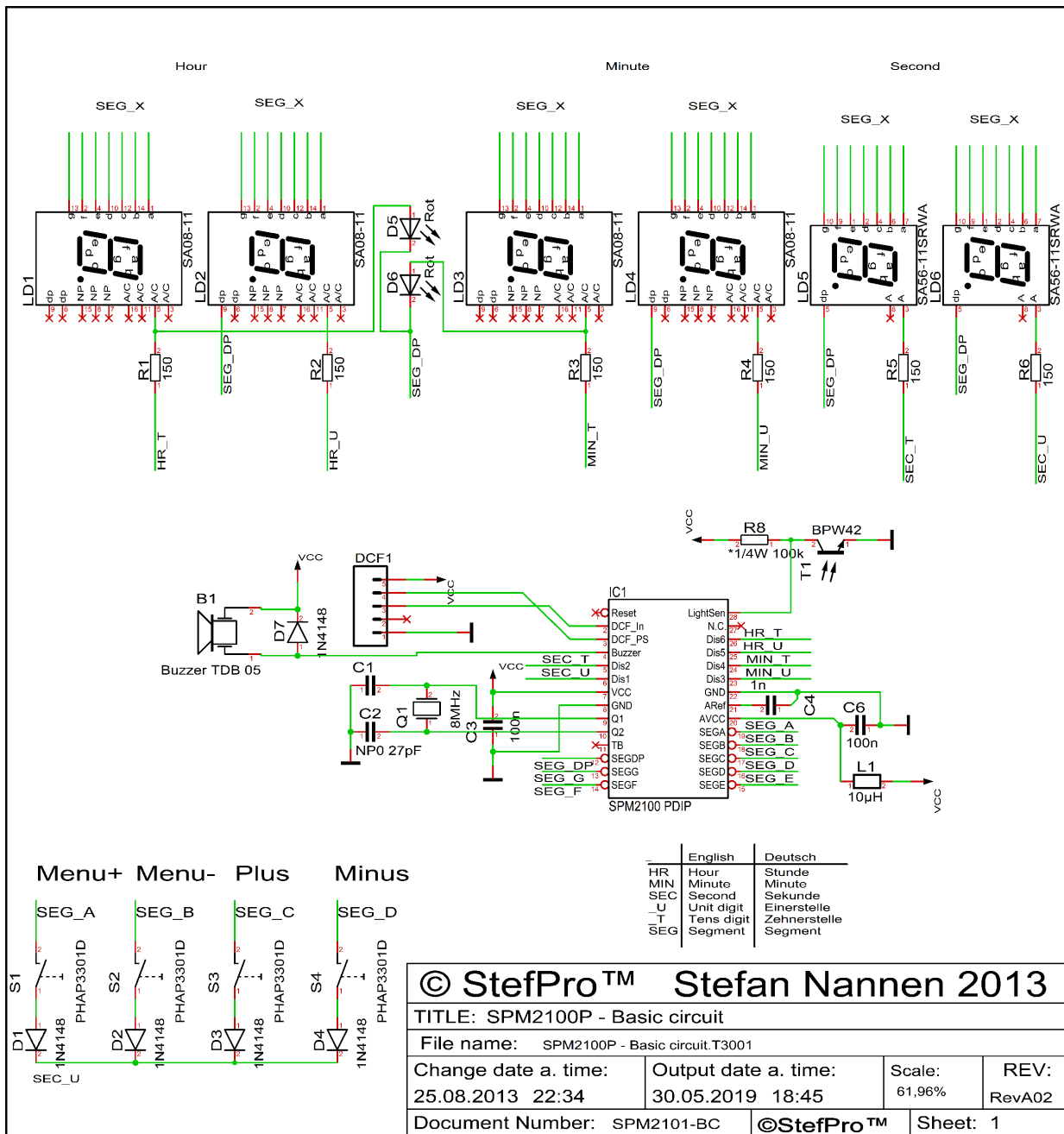
Abbildung 2: Grundschialtung vom SPM2100P
