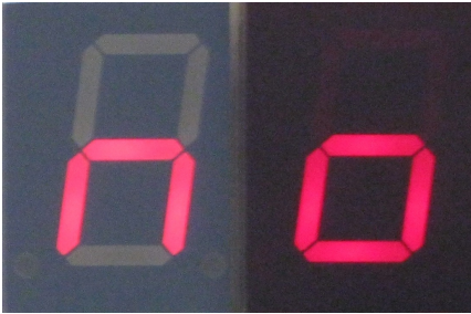
Abbildung 7: SA08-11SRWA links ohne und rechts mit Kontrastscheibe ohne Gegenlicht
