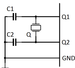
Abbildung 3: Anschluss des Quarzes
