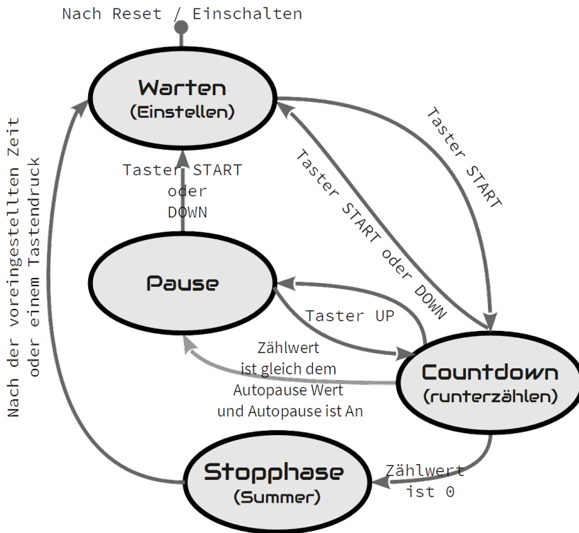
Abbildung 2: Zustandsdiagramm Countdown Betriebsarten
