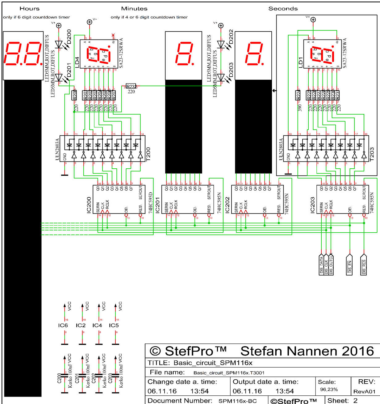
Abbildung 5: Grundschtung vom SPM1160P Teil 2
