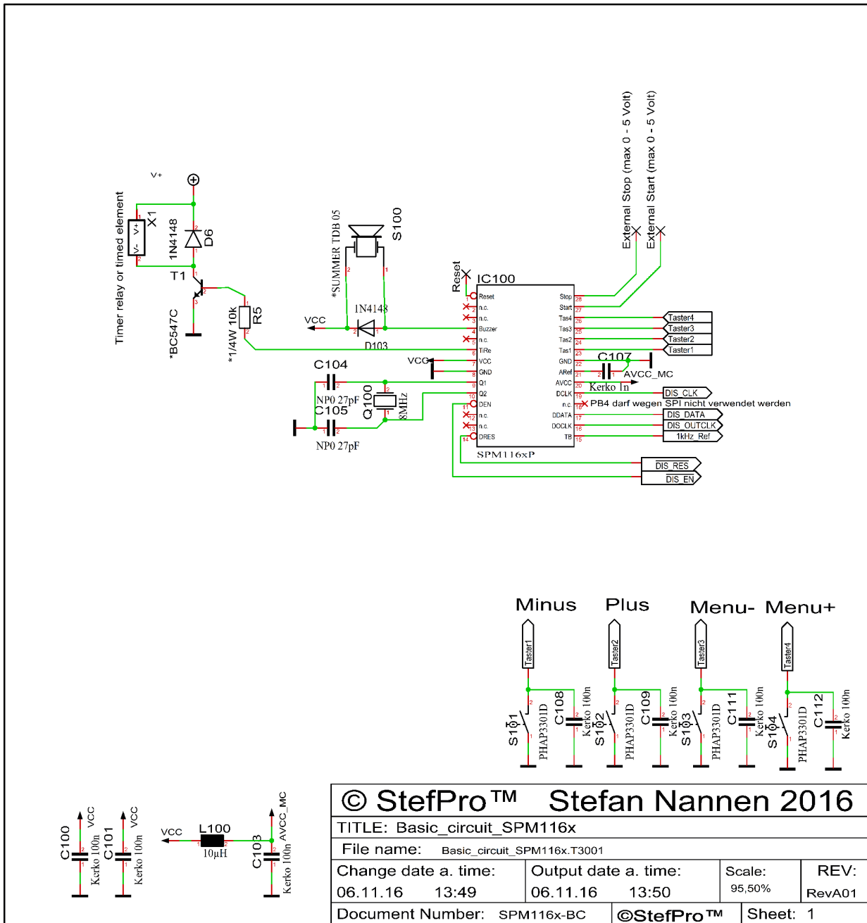
Abbildung 4: Grundschtaltung vom SPM1160P Teil 1
