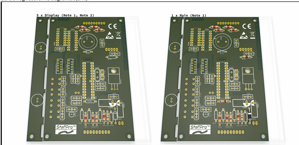
Abbildung 22: Bestückung vom SPK2141.02 Schritt 1
