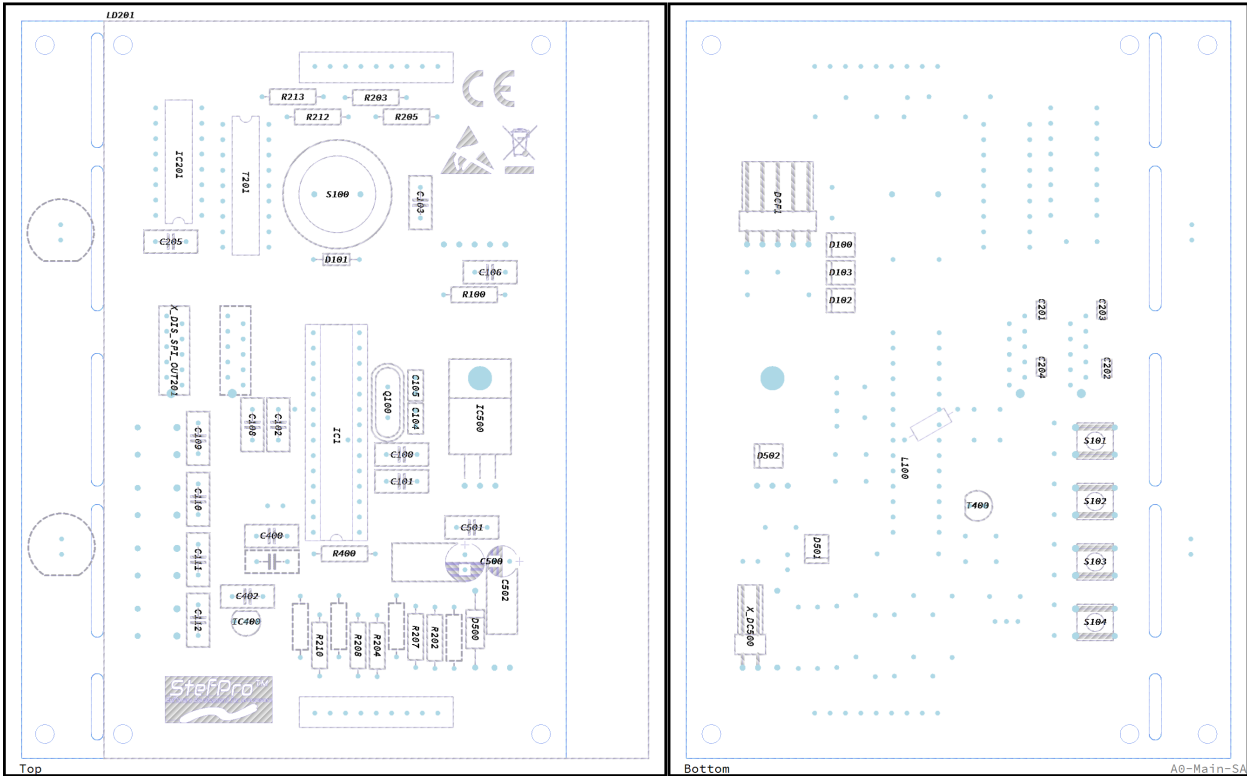
Abbildung 5: Bestückung vom SPK2141.02 Bestückungsplan mit Namen. Hauptplatine und Einerstelle von Sekunden. 1 mal zu Bestücken. Bitte Stücklisten hinweise beachten.
