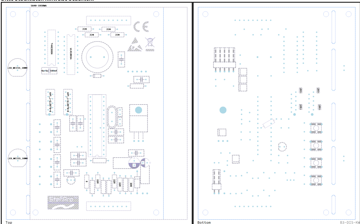
Abbildung 20: Bestückung vom SPK2141.02 7
