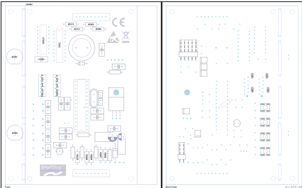
Abbildung 6: Bestückung vom SPK2141.02.1 Bestückungsplan mit Namen. Zehnerstelle von Sekunden. 1 mal zu Bestücken.
