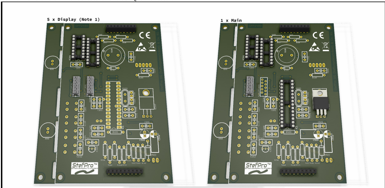
Abbildung 24: Bestückung vom SPK2141.02 Schritt 3 Als nächstes kommen die IC-Sockel für den SPM2x41P, 74HC595 und ULN2803A. Die IC's können auch direkt eingelötet werden, sollte aber nicht. Weiterhin sind die MicroMatch, Buchsenleisten und der Spannungsregler im TO220 Gehäuse an der Reihe. Note 1: Bei dem Anzeigemodul für die Zehnerstelle der Stunde muss der linke MicroMatch (grauer stecker auf dem Bild) nicht bestückt werden.
