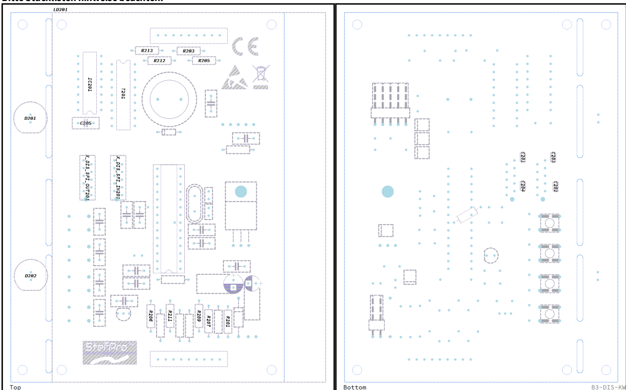
Abbildung 12: Bestückung vom SPK2141.02 7
