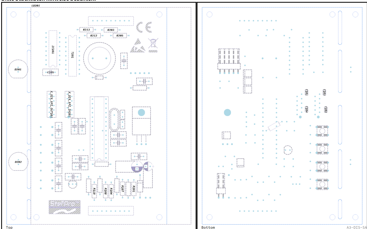
Abbildung 8: Bestückung vom SPK2141.02 3
