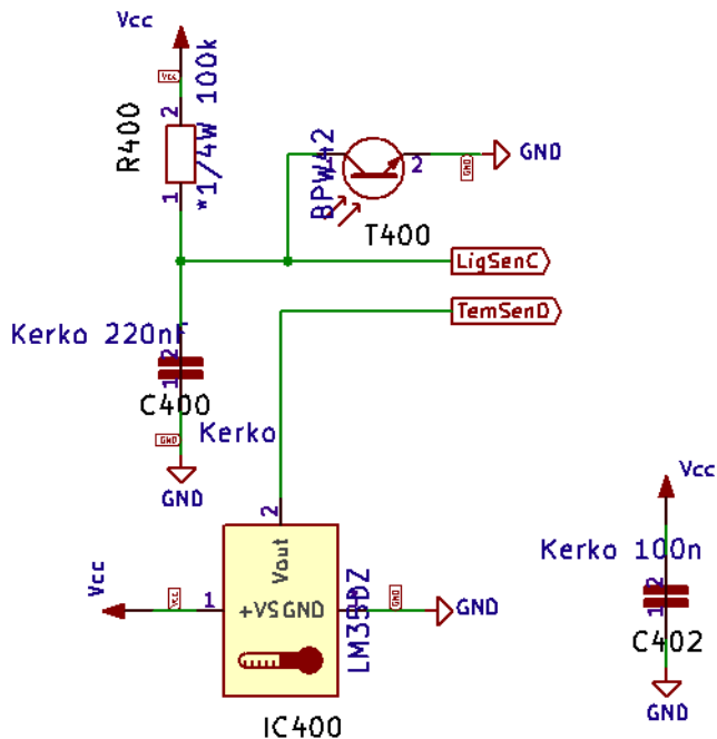
Abbildung 2: Grundschtaltung vom SPK2141.02 Teil 2
