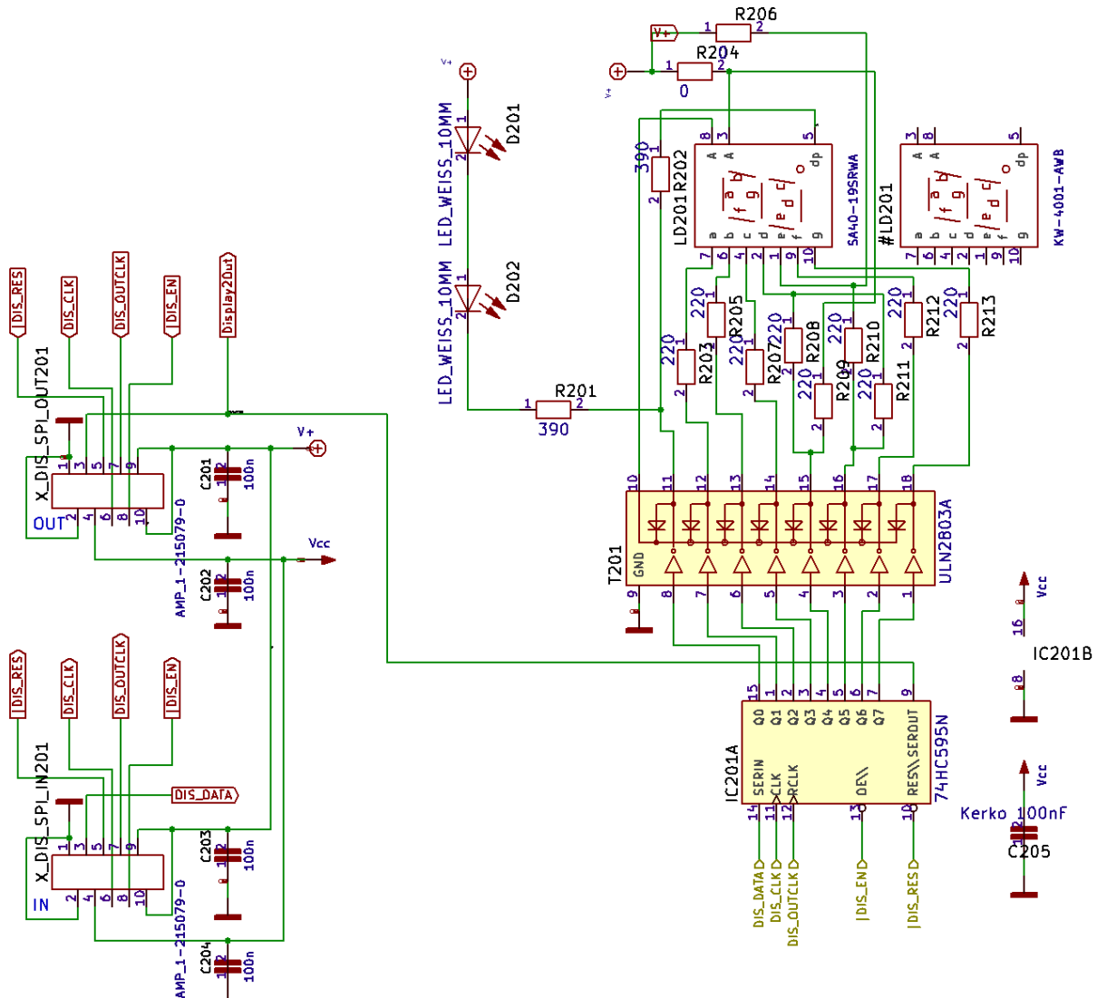
Abbildung 2: Grundschtaltung vom SPK2141.02 Teil 2
