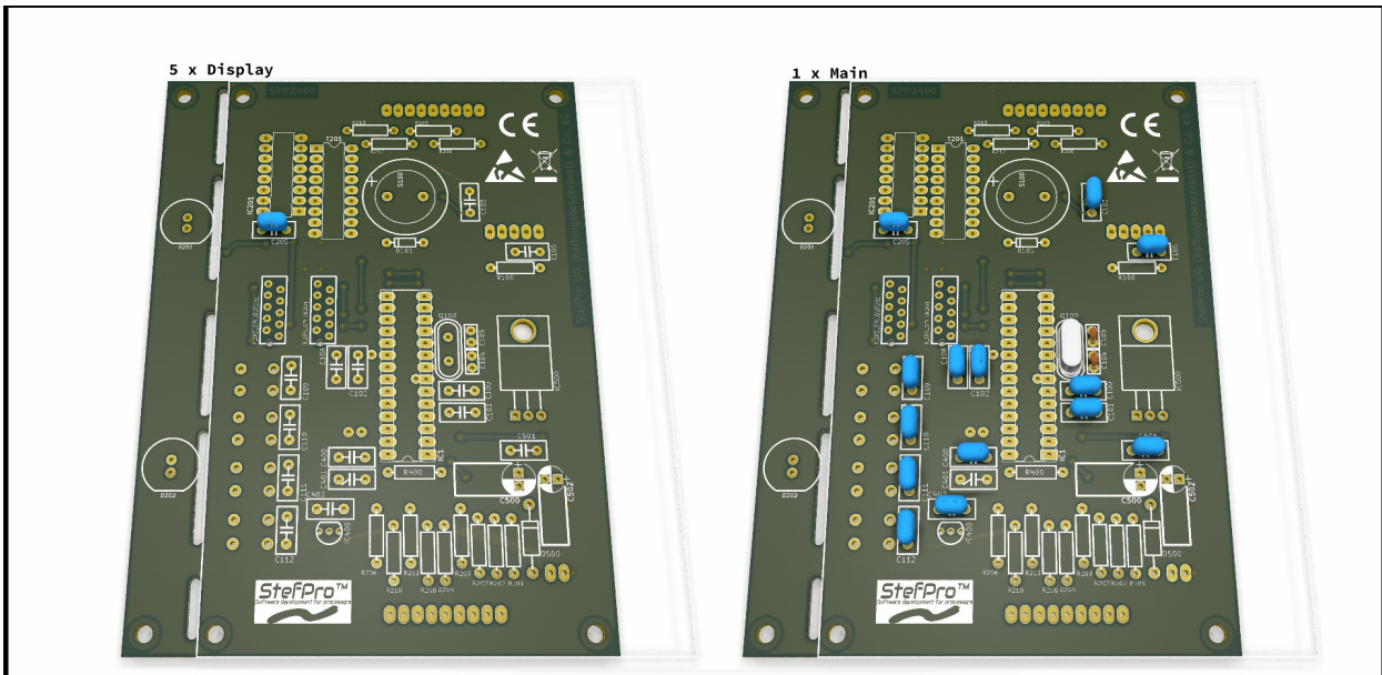
Abbildung 23: Bestückung vom SPK2141.02 Schritt 2 Nun können Sie Keramikcondensatoren und den Quarz einlöten.
