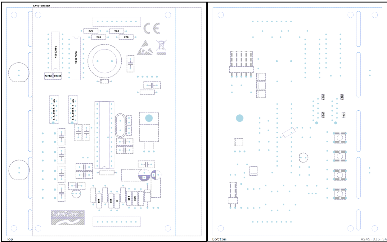
Abbildung 15: Bestückung vom SPK2141.02 2
