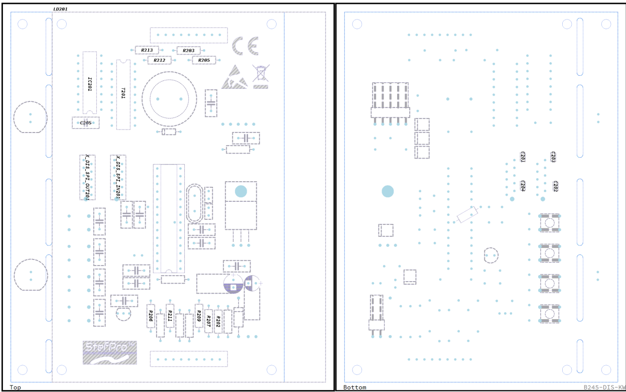
Abbildung 11: Bestückung vom SPK2141.02 6
