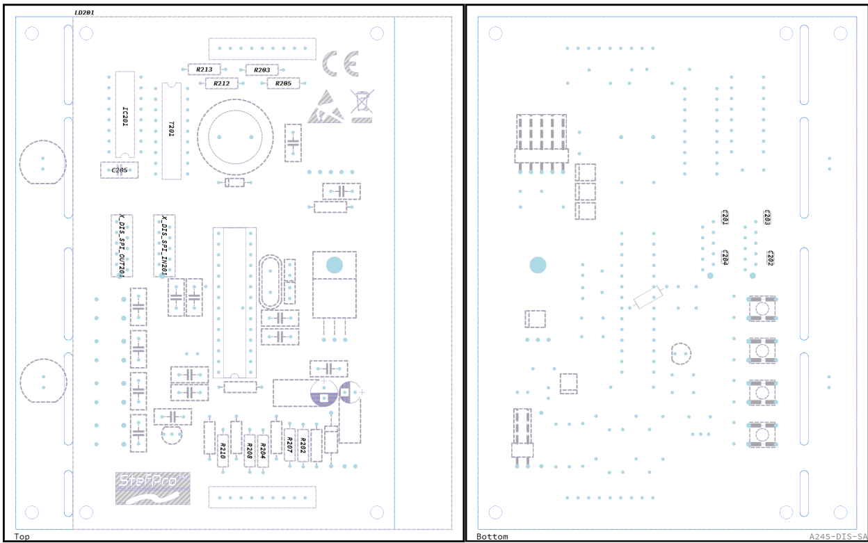
Abbildung 7: Bestückung vom SPK2141.02 2
