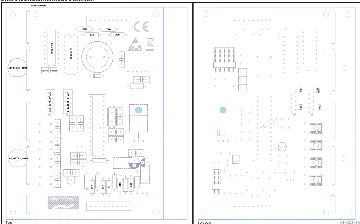
Abbildung 16: Bestückung vom SPK2141.02 3
