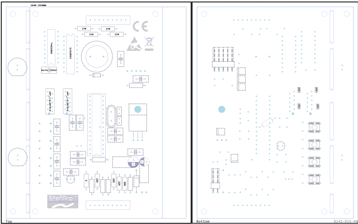
Abbildung 19: Bestückung vom SPK2141.02 6
